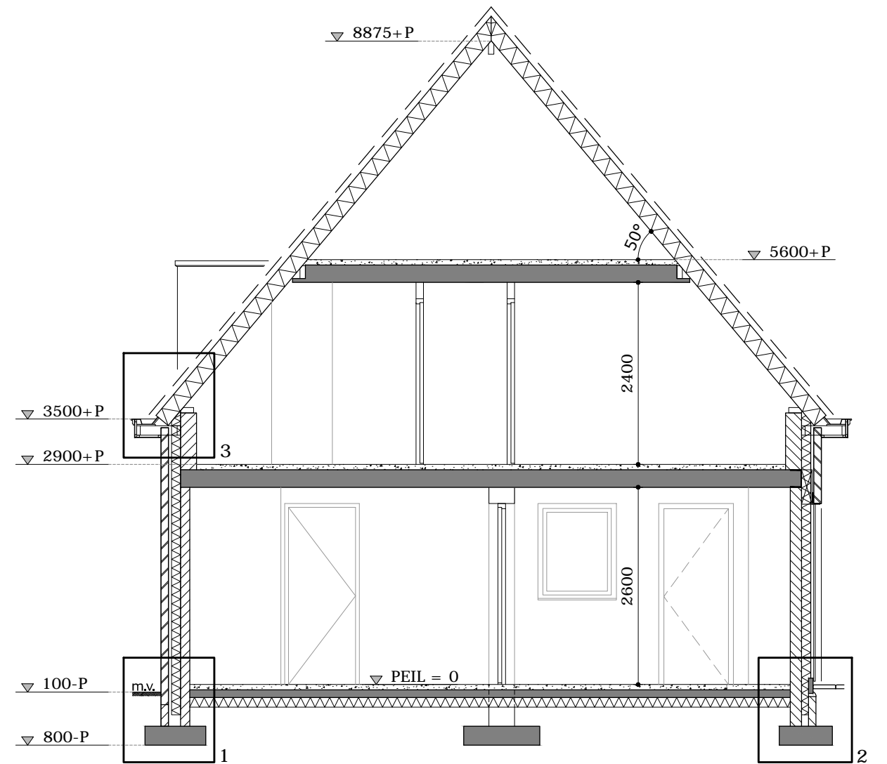
DOORSNEDE A-A
