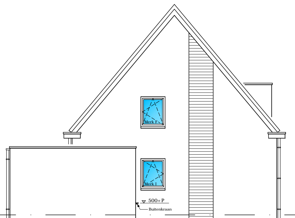
LINKER ZIJGEVEL
